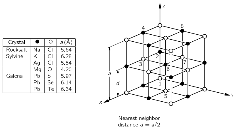
图 1.7: 食盐的晶体结构
