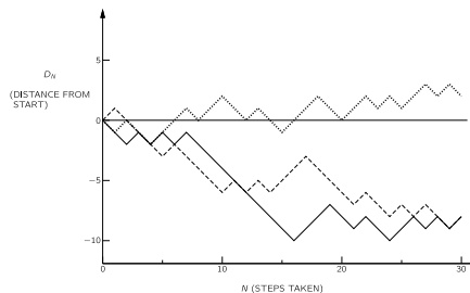
图 6.5: 无规行走取得的进度。横座标 N 表示所走的步数总数；纵座标 D_N 表示离开起点的净距离
