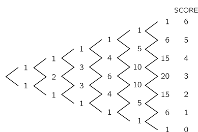
图 6.4: 抛掷六次游戏的图解
