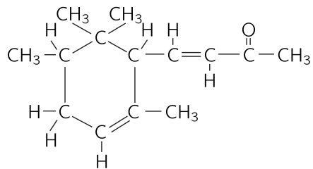
图 1.10: \alpha 鸢尾酮香料的分子结构图
