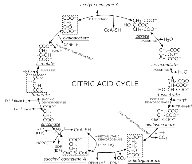
图 3.1: 克莱布斯循环
