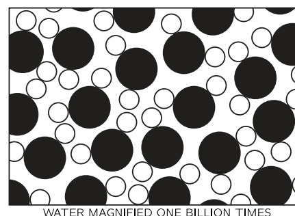
图 1.1: 放大 10 亿倍的水
