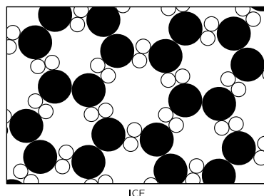
图 1.3: 冰
