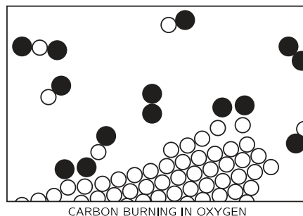
图 1.8: 碳在氧气中的燃烧
