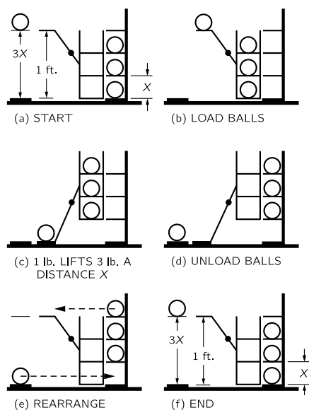
图 4.2: 一种可逆机
