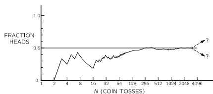
图 6.6: 获得正面的那些抛掷在某一特定次序中的比值
