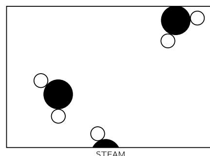
图 1.2: 水蒸气
