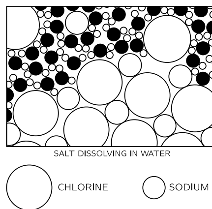
图 1.6: 盐在水中的溶解
