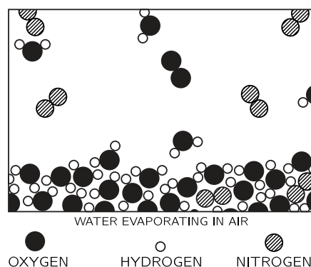
图 1.5: 空气中水的蒸发
