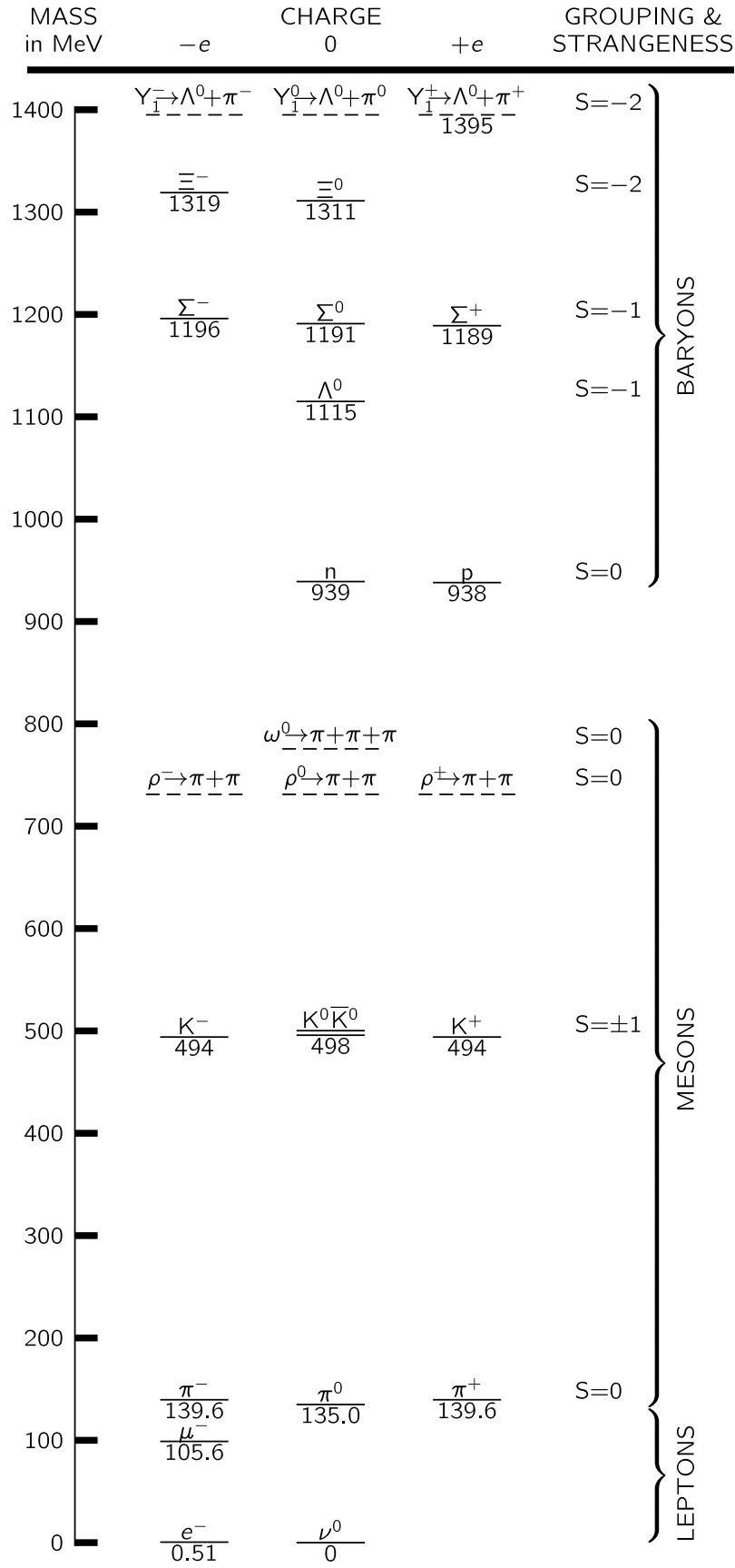
图 2.1: 基本粒子
