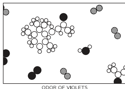
图 1.9: 空气中的紫罗兰香气分子
